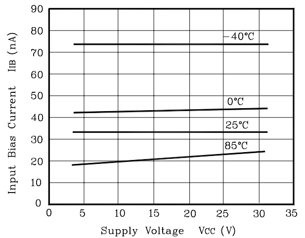
Fig. 2 V_{CC} - I_{IB}
