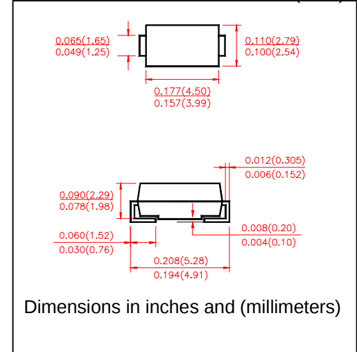
DO-214AC(SMA)
