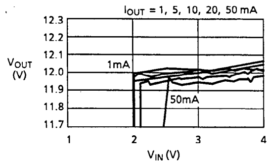
(b) V_{\text{IN}}-V_{\text{OUT}}
