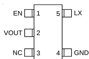
SOT-23-5
