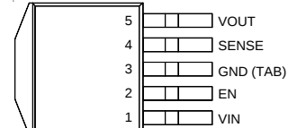
TO-263-5 RT9172S-□□xM5
