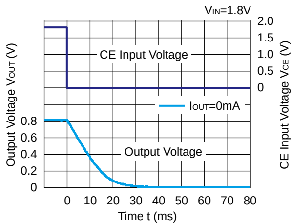
RP110x08xB
