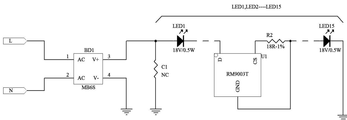
图 1 系统应用原理图
