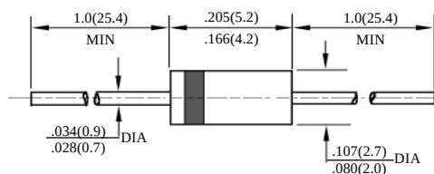
DO – 41
