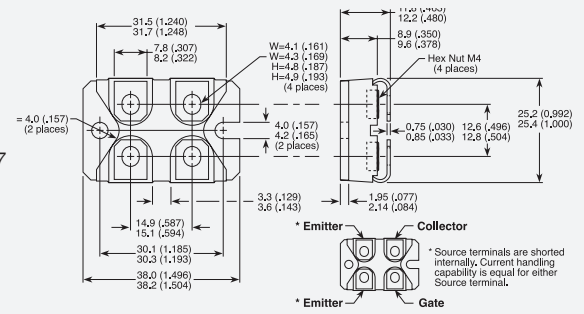
SOT-227
