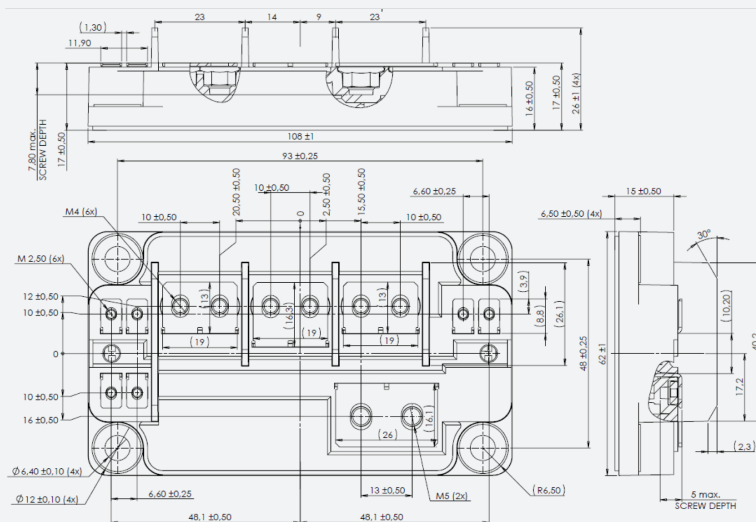
SP6LI
