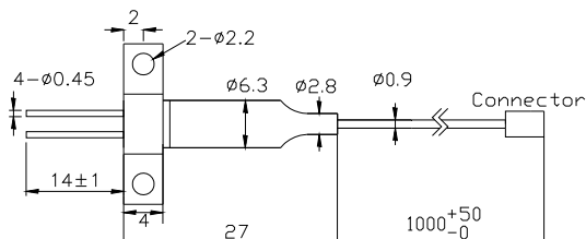
Horizontal Flange
