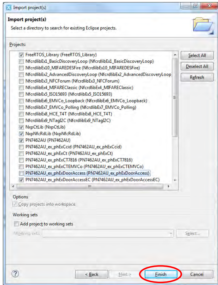
Fig 20. Select project
