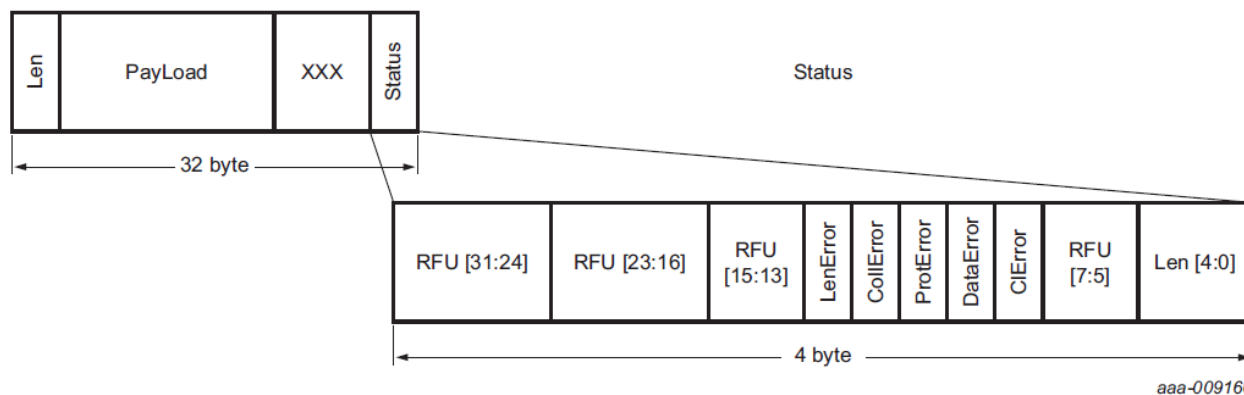
Fig 29. RXMultiple data format
