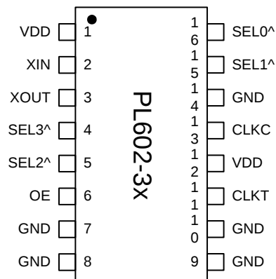
TSSOP-16L
