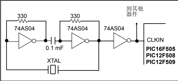
图 7-4: 外部串联谐振器的晶振电路
