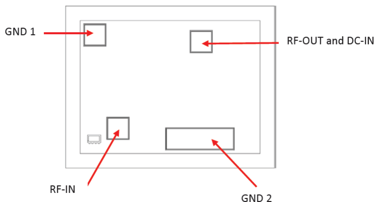
Fig 2. Die Layout
