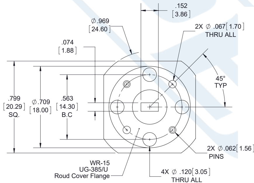
VIEW A-A
