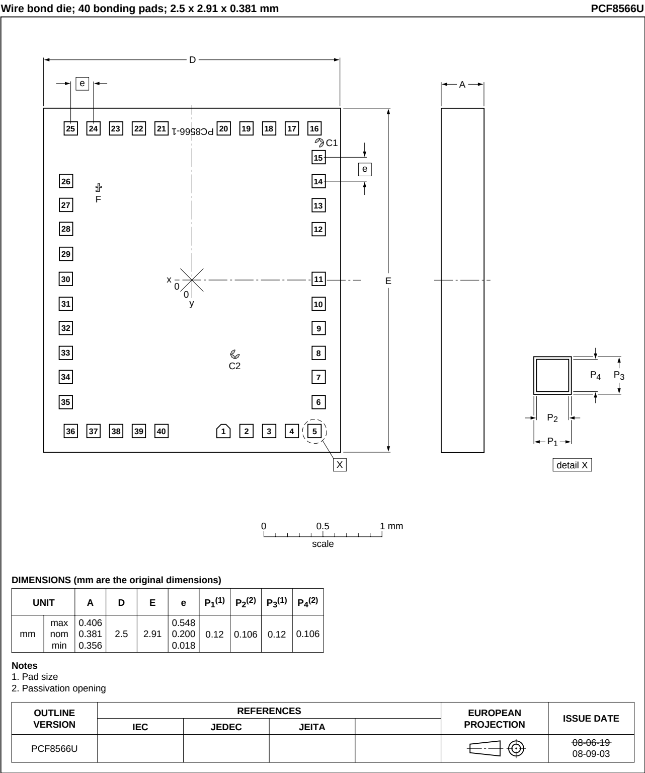
Fig 31. Bare die outline PCF8566U
