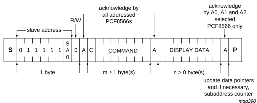
Fig 17. I 2 C-bus protocol
