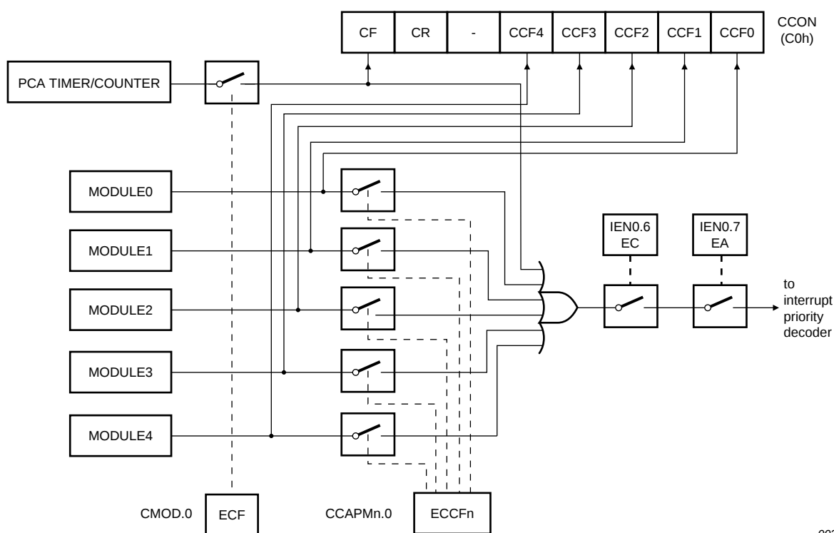
Fig 27. PCA interrupt system
