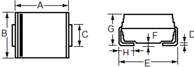
SMB (DO-214AA)
