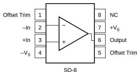
SO-8
