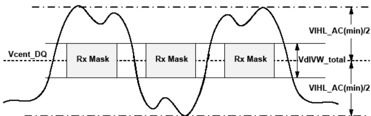
DQ VIH AC definition (for each input pulse)
