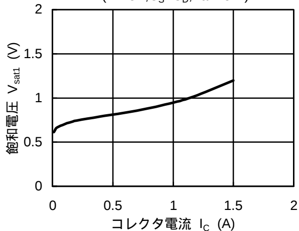
飽和電圧1対コレクタ電流特性例 ( V^+=5V, C_S=C_D, T_a=25^\circ\text{C} )
