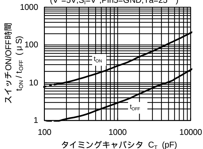
スイッチON/OFF時間対タイミングキャパシタ特性例 ( V^+=5V, S_I=V^+, \text{Pin5=GND}, T_a=25^\circ\text{C} )
