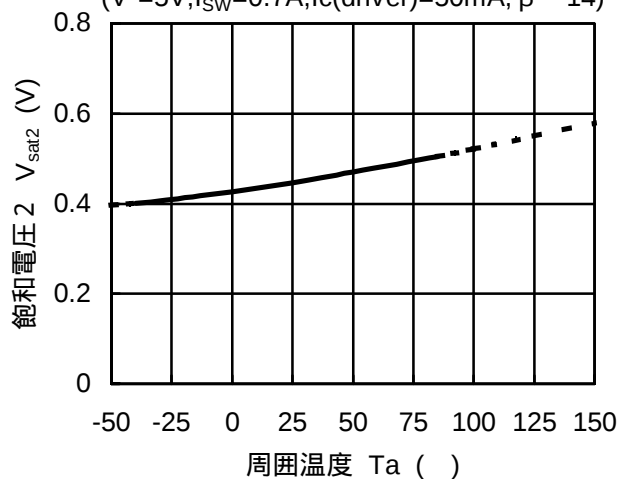
飽和電圧 2 温度特性例 ( V^+=5V, I_{SW}=0.7A, I_c(driver)=50mA, \beta=14 )
