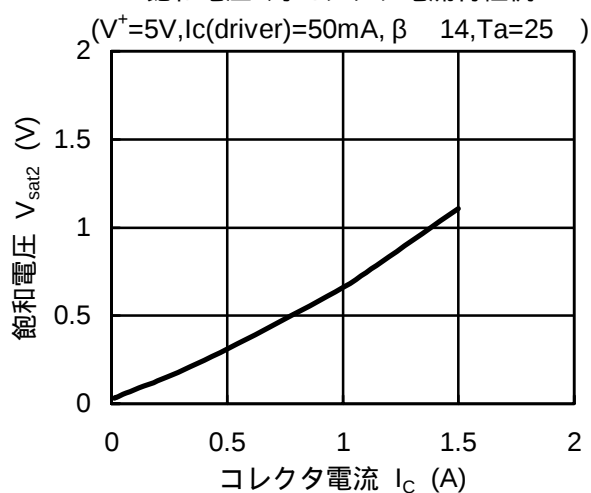
飽和電圧2対コレクタ電流特性例
