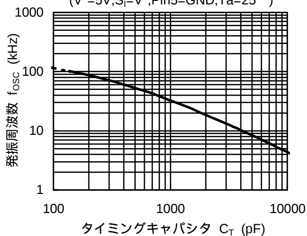
発振周波数対タイミングキャパシタ特性例 ( V^+=5V, S_I=V^+, \text{Pin5=GND}, T_a=25^\circ\text{C} )
