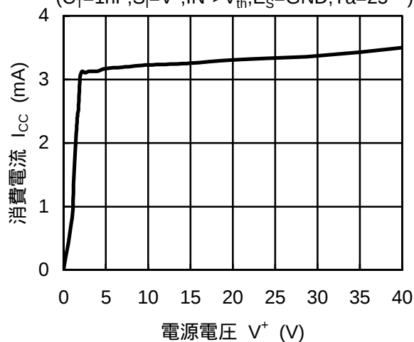
消費電流対電源電圧特性例 ( C_T=1nF, S_I=V^+, I_{N^+}>V_{th}, E_S=GND, T_a=25^\circ\text{C} )
