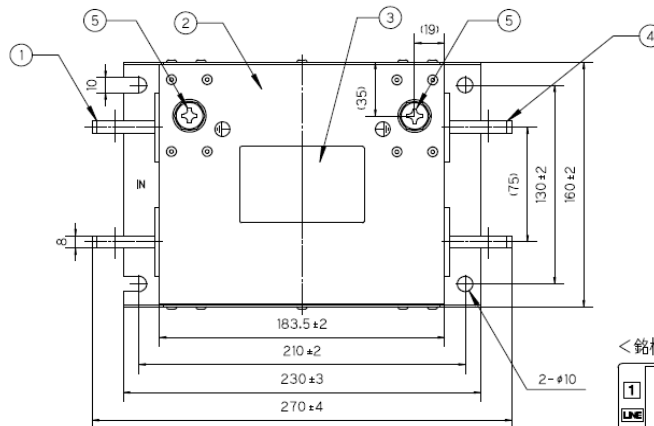
fig.1 (300, 600A)
