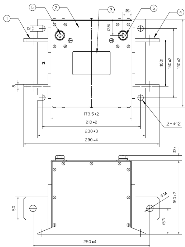
fig.2 (1000A)
