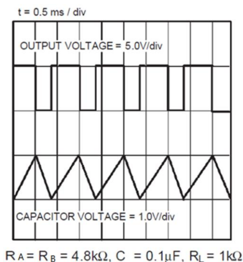
图 6 非稳态波形图
