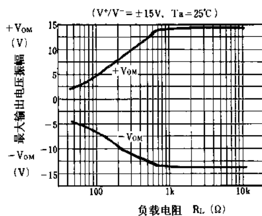
最大输出电压振幅与负载电阻
