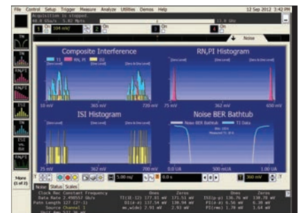
EZJIT Complete.
