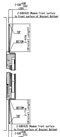
SECTION YY-YY SCALE 5:1
