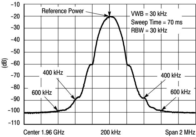
Figure 16. EDGE Spectrum
