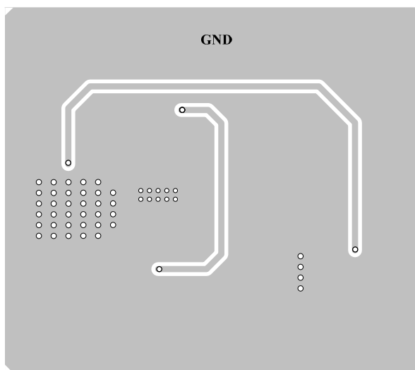
Bottom Layer
