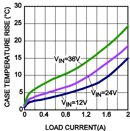
Thermal Rise
