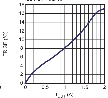
Case Thermal Rise
