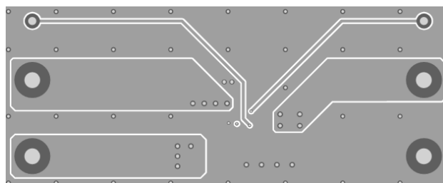
Inner Layer 2
