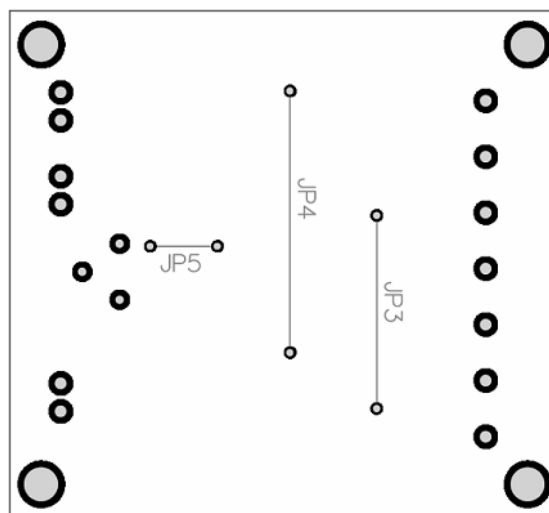
Top Layer
