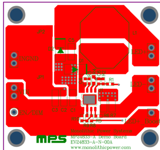
Top Layer
