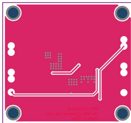
Bottom Layer
