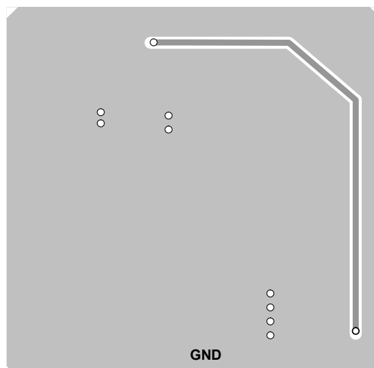
Bottom Layer
