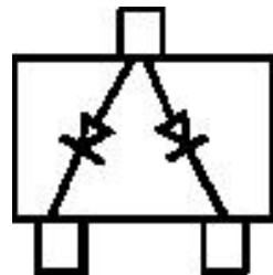
SOT-23 封装内部结构
