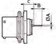
Type 7 Jam nut receptacle
