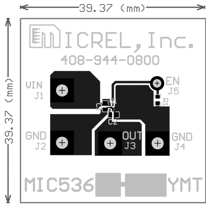
Top Layer
