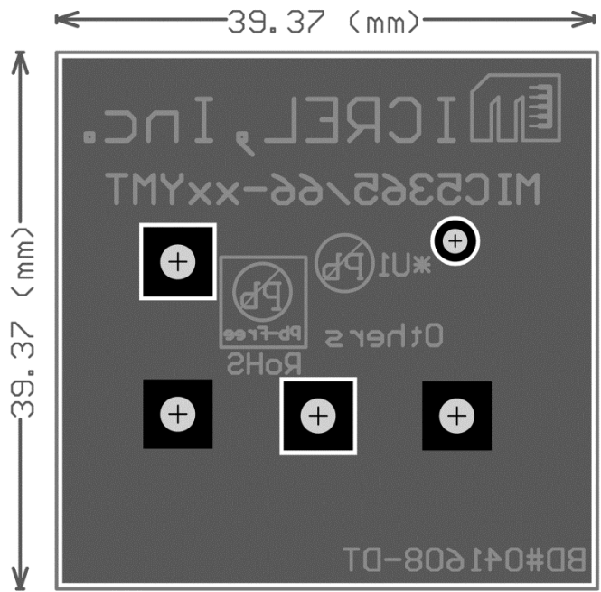
Bottom Layer
