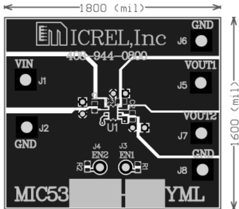
Top Layer
