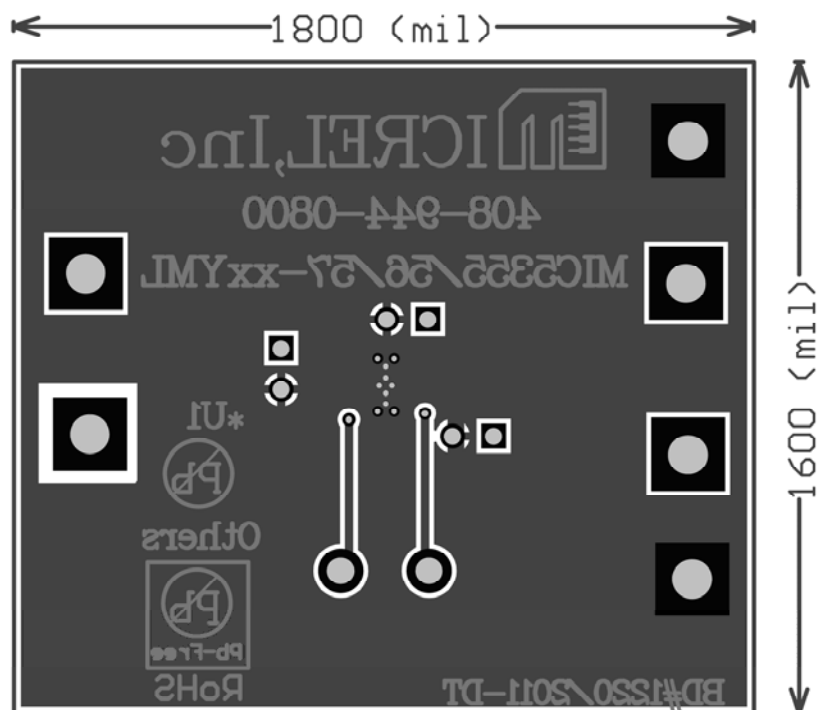
Bottom Layer
