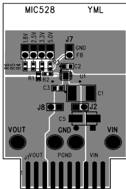
Top Layer
