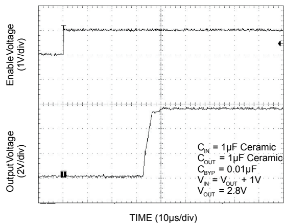
Enable Turn-On
