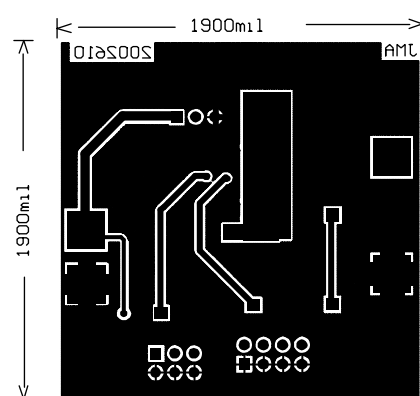
Figure 5e. Bottom Layer
