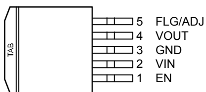
TO-263-5 (U)
