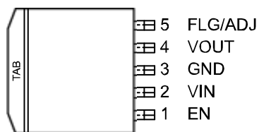
S-PAK-5 (R)
