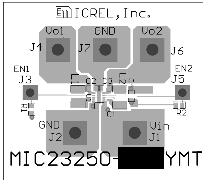
Top Layer
