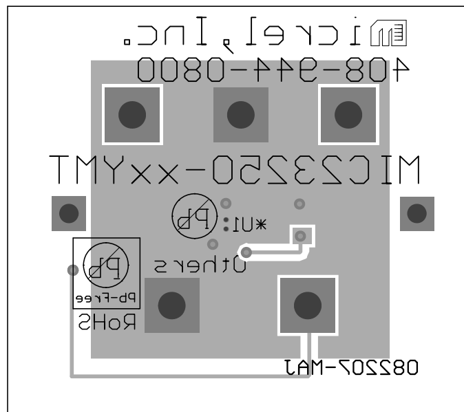
Bottom Layer
