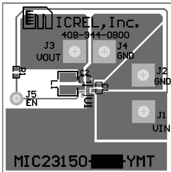
Top Layer
