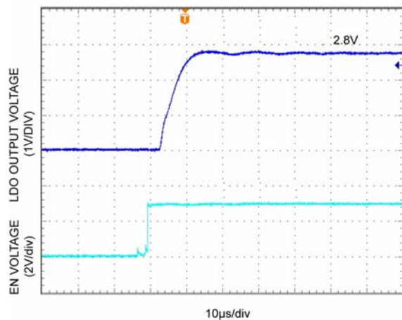
LDO Enable
