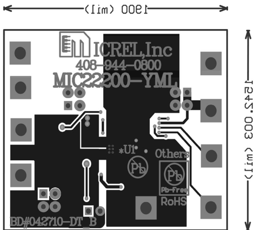
Bottom Layer
