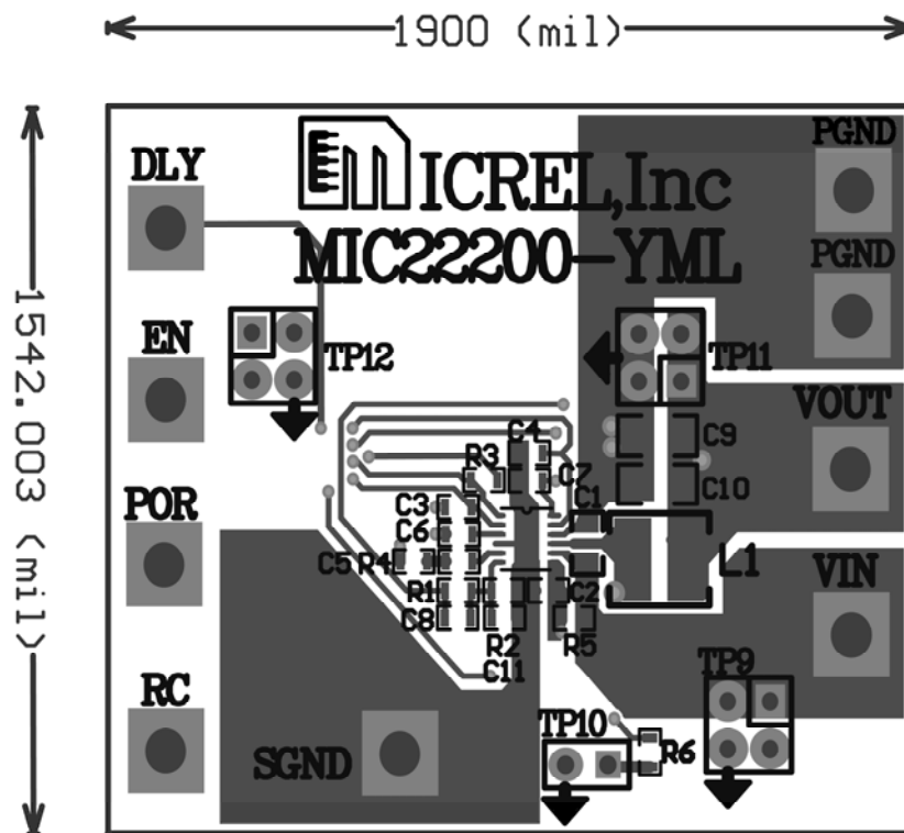
Top Layer
