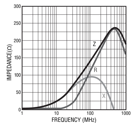
MH 1608- 151Y
