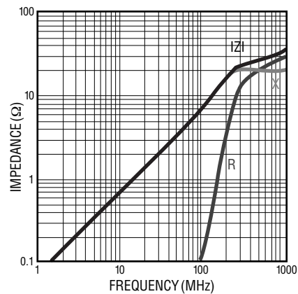
MH 2029- 070Y
