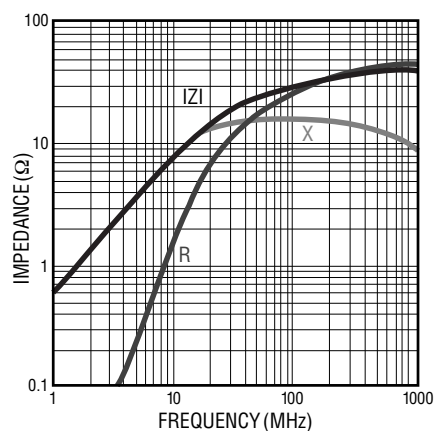
MH 2029- 300Y
