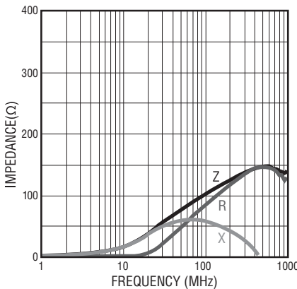
MH 1608- 101Y
