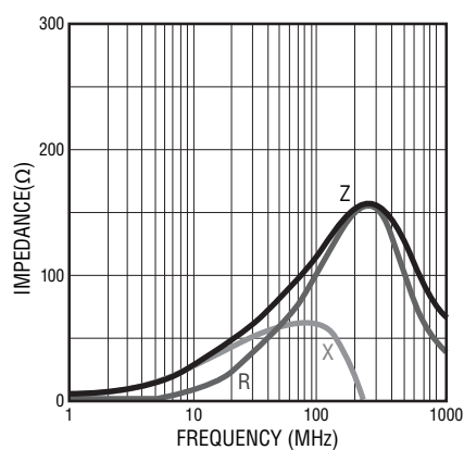
MH 2029- 121Y
