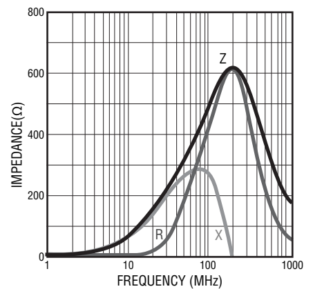
MH 1608- 471Y
