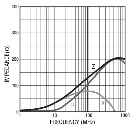
MH 2029- 151Y
