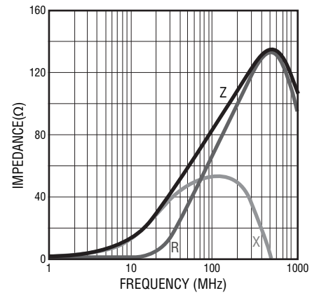
MH 1608- 800Y
