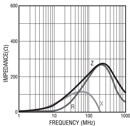
MH 2029- 221Y
