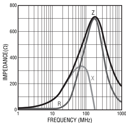
MH 1608- 601Y
