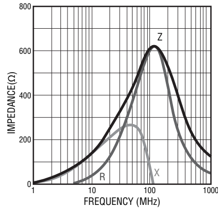
MH 2029- 601Y
