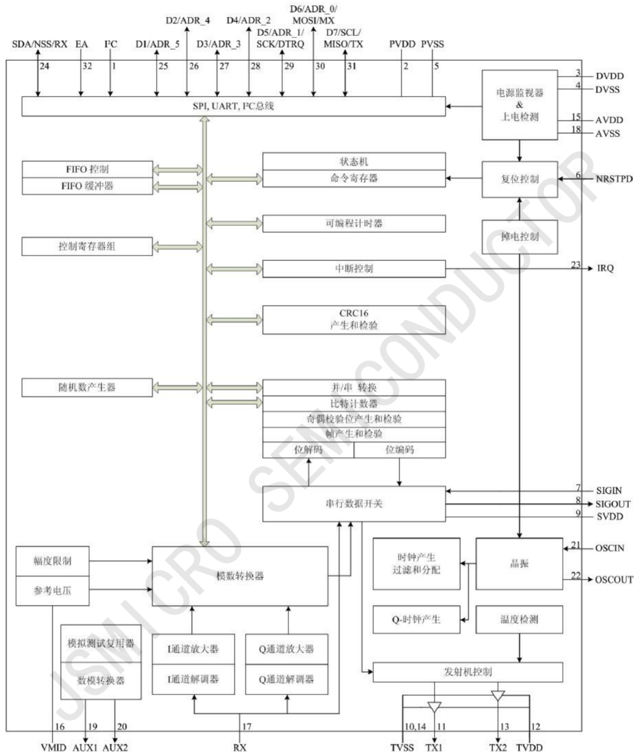
图 2 功能框图
