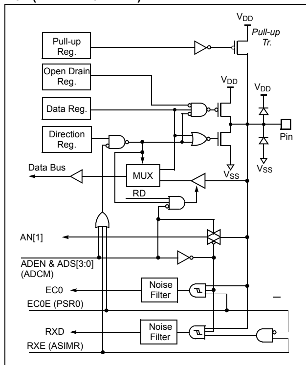
R04 (AN4 / EC0 / RXD)
